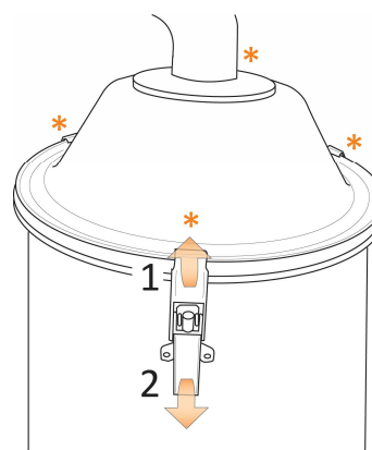
Obr 4-6: Osazení krytu
